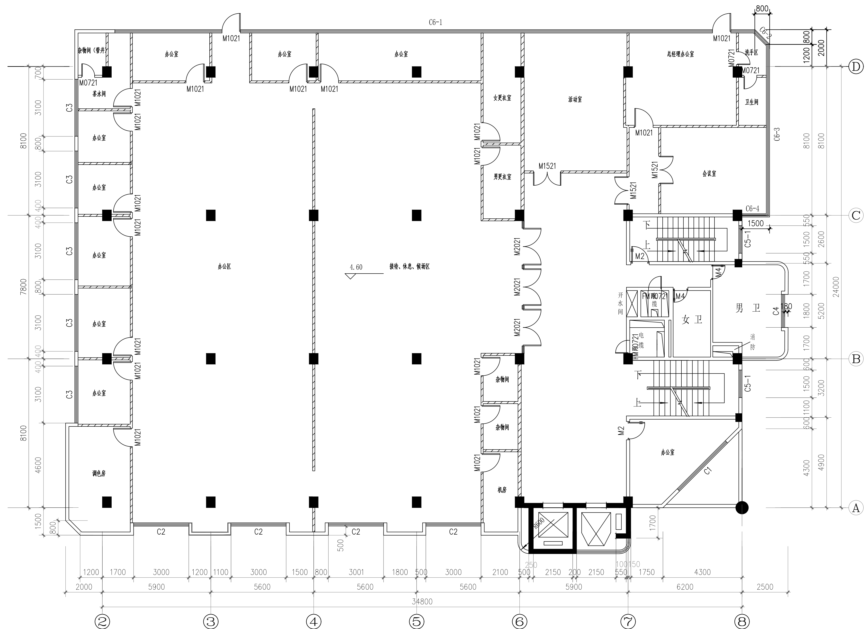
二层平面图 1:100
